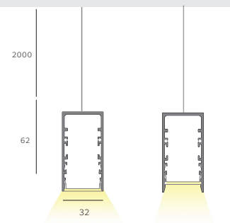
Diffusore complanare | Complanar diffuser Diffusore arretrato | Backward diffuser
