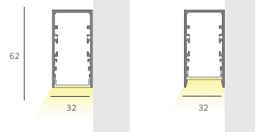
Diffusore complanare | Coplanar diffuser
