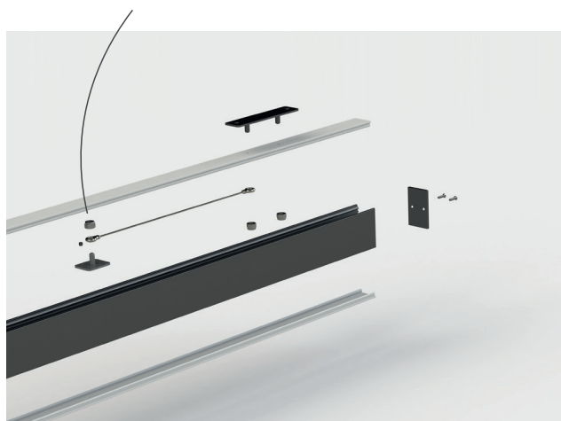
KIT DI SICUREZZA / SAFETY KIT MOUNTING
